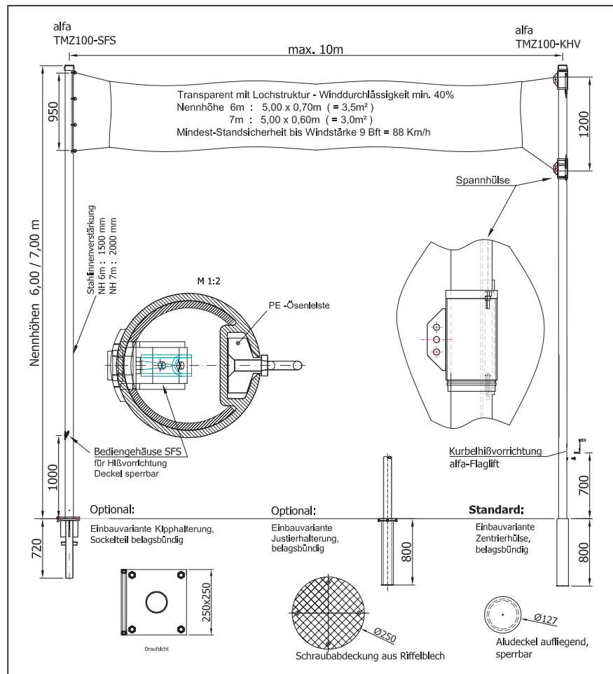
Hissbare Ösenleiste alfa TMZ100-SFS
