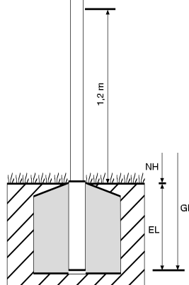
Passform-Bodenhülse für Ø 90 mm
