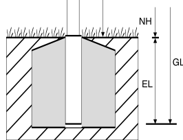
Passform-Bodenhülse für Ø 90 mm
