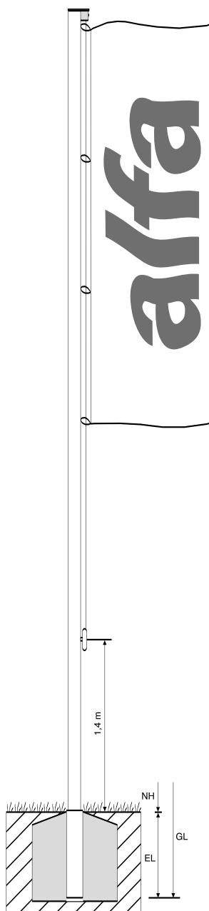
Passform-Bodenhülse für Ø 90 mm
